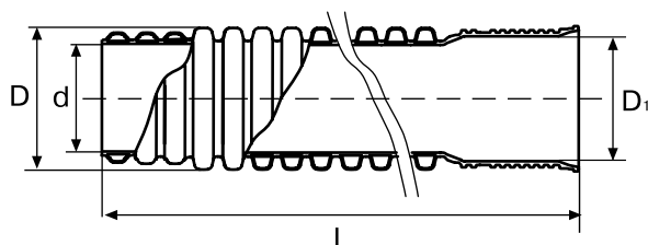
Труба ИКАПЛАСТ с раструбом исп. 2 (с уменьшенной высотой гофра в месте соединения с раструбом) Класс жесткости SN8, SN10 и SN16
